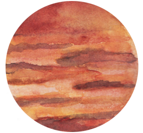
Júpíter
