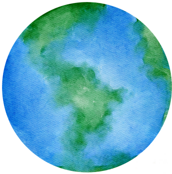
Jörðin
